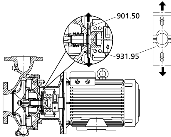
Afb. 10: Borgplaatjes verwijderen
