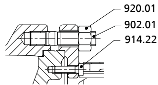
Afb. 13: Bevestiging geklemd huisdeksel
