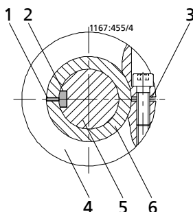
Afb. 9: Asstomp van de motor op de as monteren
