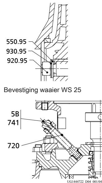
Ontluchtingsventiel 5B
