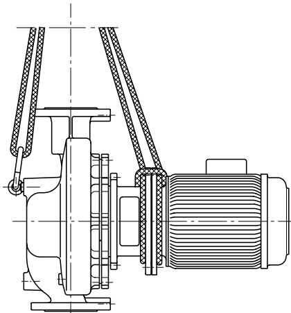
Afb. 1: Pompaggregaat transporteren
