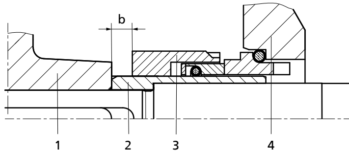
Afb. 8: Mechanische asafdichting inbouwmaat b
