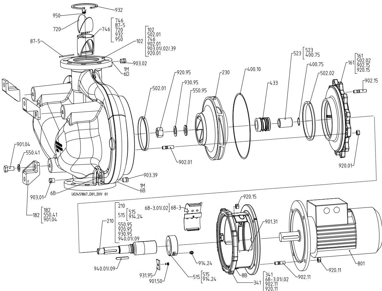
Afb. 11: Uitvoering met geschroefd huisdeksel
