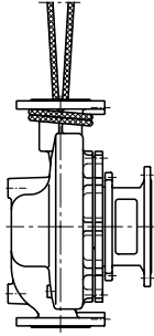
Afb. 2: Pomp transporteren
