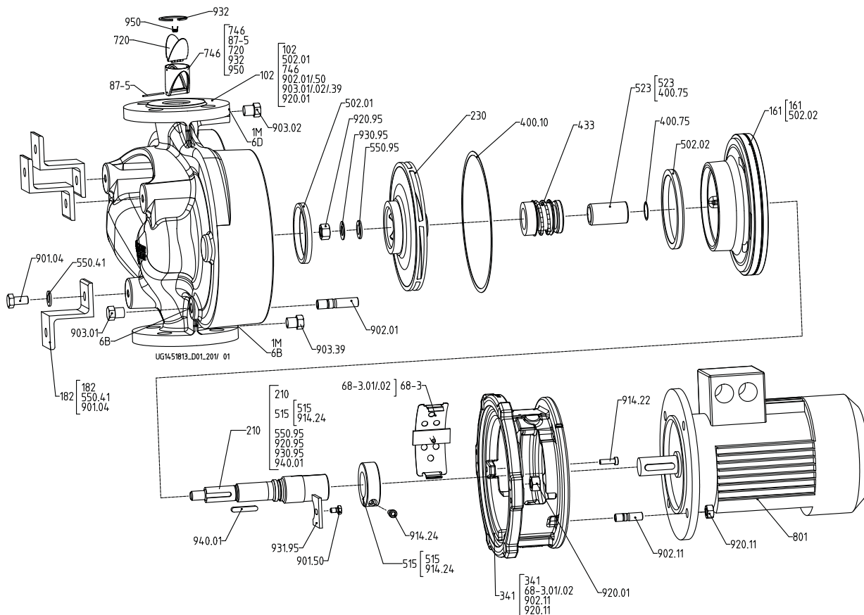
Afb. 12: Uitvoering met enkelwerkende mechanische asafdichting en geklemd huisdeksel
